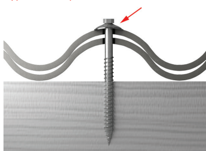
rys.25. Tradycyjny system montażowy Cembrit przykręcony poprawnie. Podkładka aluminiowa nie może zostać zdeformowana od zbyt dużej siły docisku.
