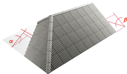
rys. 37. Nachylenie połaci dachowych przecinających się w narożu.
