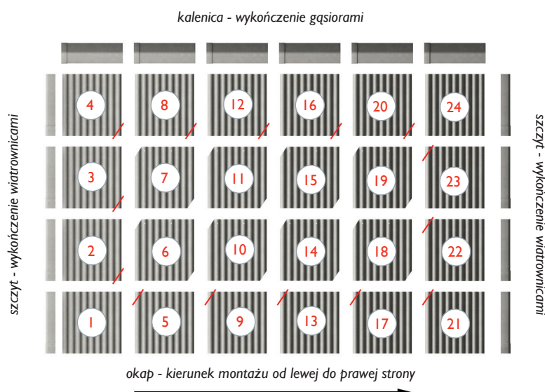
rys. 23. Prawidłowa kolejność układania płyt EuroFala NO/WO zgodnie z numeracją od 1 do 24.
