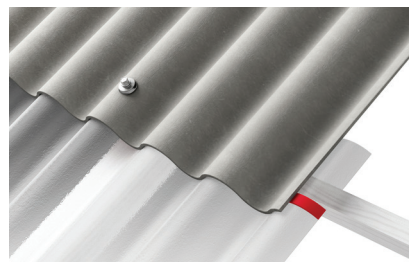
rys.28. Zakład poprzeczny płyty świetlikowej Eurolux, zamontowanej pod płytą falistą EuroFala.
