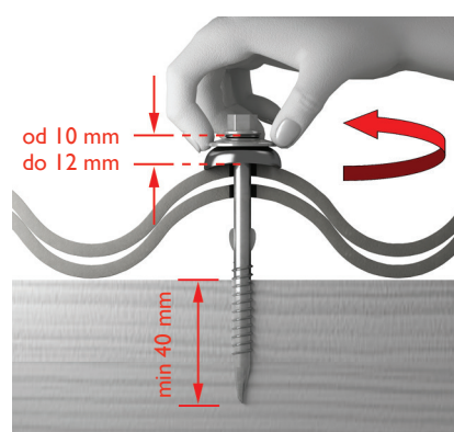
rys.26. System montażowy Quick Fix do konstrukcji drewnianej przykręcony poprawnie. Prawidłowość przykręcenia systemu montażowego ocenia się wizualnie oraz próbując okrócić stalową podkładkę dociskową wokół osi wkrętu. Jeżeli nie jest to możliwe to znaczy, że system montażowy jest przykręcony zbyt mocno i musi zostać poluzowany. Wkręt musi być wkręcony do łaty/płatwi na głębokość min. 40 mm.
