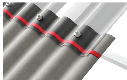
rys.29. Zakład poprzeczny płyty świetlikowej Eurolux, zamontowanej nad płytą falistą EuroFala.
