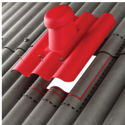
rys. 10. Komin wentylacyjny sanitarny HV 110 - powierzchnia wentylacji 90 cm²
