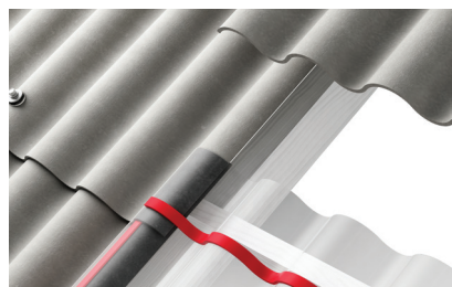
rys.31. Zakład podłużny i poprzeczny płyty świetlikowej Eurolux, zamontowanej przy płytach EuroFala.
