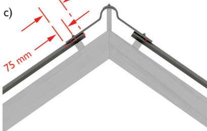
rys.34. Sposób wykończenia kalenicy: a - gąsiosem kątowym b - gąsiosem konikalnym / stożkowym c - gąsiosem zawiasowym płaskim
