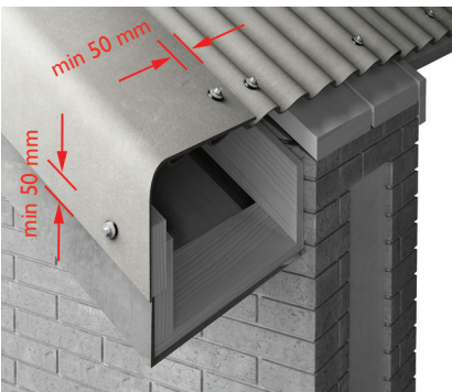
rys.39. Montaż wiatrownicy o prostym ramieniu.
