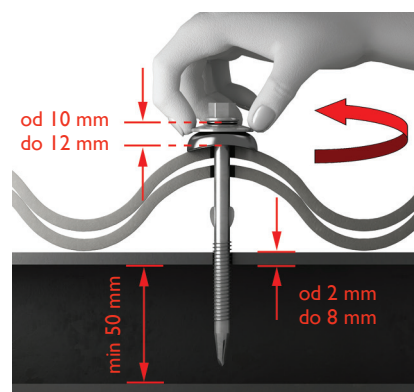
rys.27. System montażowy Quick Fix do konstrukcji stalowej przykręcony poprawnie. Prawidłowość przykręcenia systemu montażowego ocenia się wizualnie oraz próbując okrócić stalową podkładkę dociskową wokół osi wkrętu. Jeżeli nie jest to możliwe to znaczy, że system montażowy jest przykręcony zbyt mocno i musi zostać poluzowany. Można go stosować przy grubości stali od 2 mm do 8 mm. Odległość wewnętrzna pomiędzy ściankami płatwi stalowych powinna wynosić minimum 50 mm. Systemy montażowe Quick Fix do konstrukcji stalowej zostały wyposażone w dodatkowy frez na ostrzu wierzącym. Rozwierca on wstępny otwór montażowy w płycie, a następnie wyłamuje się podczas wiercenia w konstrukcji stalowej.
