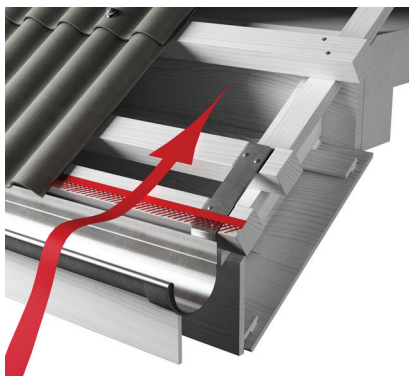
rys.5. Grzebień okapowy - powierzchnia wentylacji na 1 mb okapu: płyta W130-9 (B59) - 120 cm 2 ; płyta W177-6.5 (B65) - 200 cm 2
