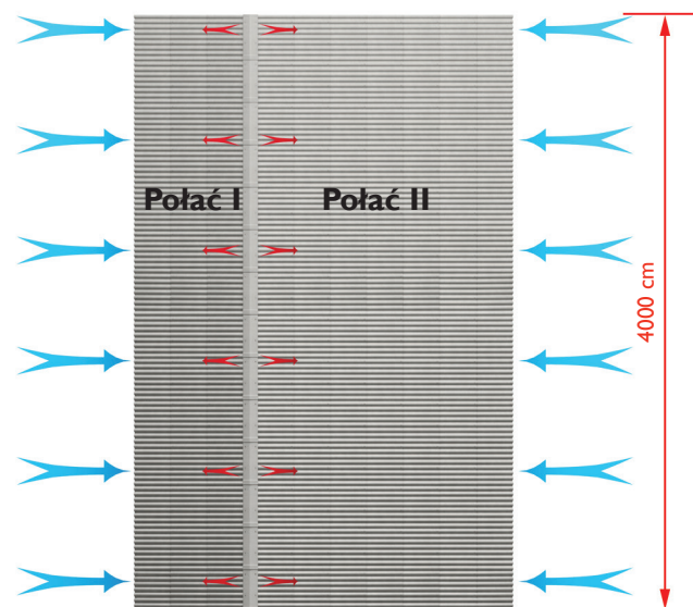
rys.12. Rysunek do przykładowych obliczeń powierzchni otworów wentylacyjnych - rzut i przekrój dachu. Niebieskie strzałki - powierzchnia otworów wentylacyjnych wlotowych w okapie. Czerwone strzałki - powierzchnia otworów wentylacyjnych wylotowych w kalenicy.
