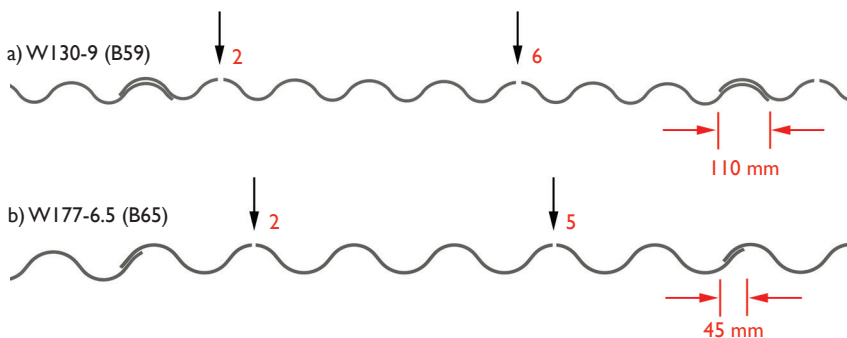
rys. 16a. Miejsca wykonania otworów montażowych dla krycia rozpoczętego z lewej strony połaci dachowej - EuroFala W130-9 (B59). rys. 16b. Miejsca wykonania otworów montażowych dla krycia rozpoczętego z lewej strony połaci dachowej - EuroFala W177-6.5 (B65).
