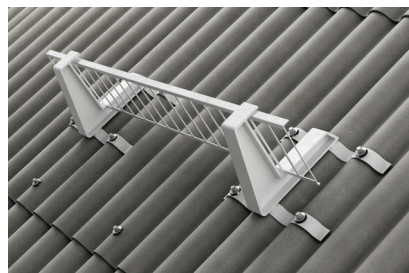
rys.49. Zabezpieczenie przeciwśniegowe.
