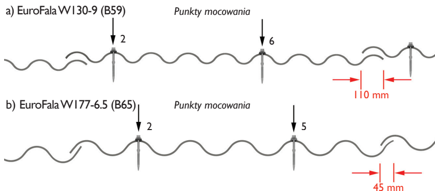
rys.24a. Punkty mocowań płyty EuroFala W130-9 (B59) na połaci dachowej znajdują się na szczytach 2 i 6 fali. Rysunek przedstawia krycie połaci dachowej od lewej do prawej strony.
