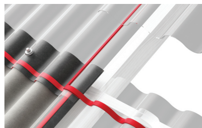
rys.32. Zakład podłużny i poprzeczny między dwiema płytami świetlikowymi Eurolux.
